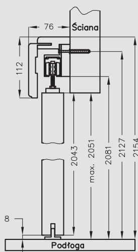
NS - przekrój pionowy
