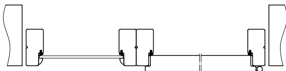
Sugerowany sposób połączenia naświetli na profilu ościeżnicy stałej
