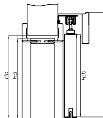
drzwi przesuwne – system naścienny z zabudową tunelową ZN OK6
