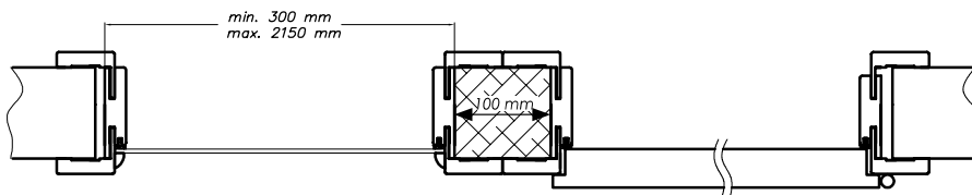
Sugerowany sposób połączenia naświetli na profilu ościeżnicy DIN przy użyciu klocków montażowych
