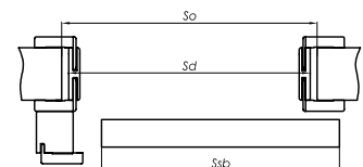
drzwi przesuwne – system naścienny z zabudową tunelową ZN OK6
