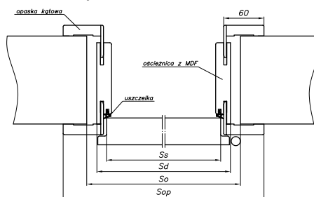
Regulowana SYSTEM DIN
