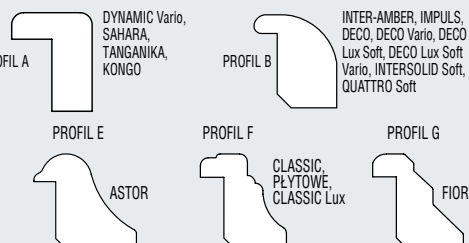
PROFILE RAMEK DO SKRZYDEŁ SZKLOWYCH
