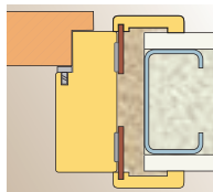
Montaż na piankę w ścianie z płyty kartonowo-gipsowej
