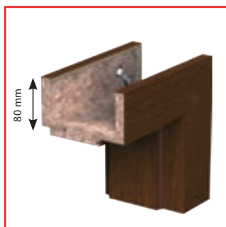
profil ościeżnicy - szeroka listwa 80 mm
