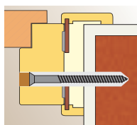
Montaż na piankę i kotwy w ścianie murowanej
