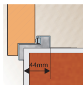
Ościeżnica kątowa mała
