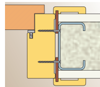
Montaż na wkręty w ścianie z płyty kartonowo-gipsowej
