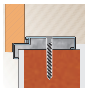
Ościeżnica kątowa duża montaż na dyble
