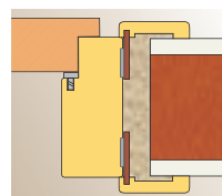
Montaż na piankę w ścianie murowanej
