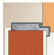
AGAT Montaż bez dodatkowych elementów kotwiących
