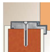
OPAL Montaż na dyble.
